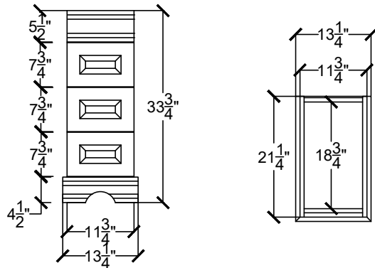
H-ARTS 1222-3D-____-____-____
