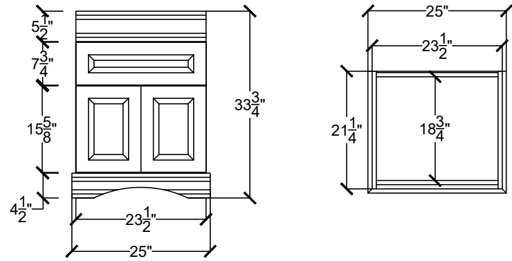
H-ARTS 2422-1D-____ - ____ - ____
