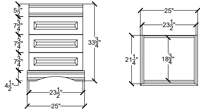
H-ARTS 2422-3D-____ - ____ - ____
