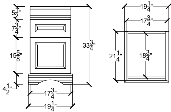
H-ARTS 1822-1D-____ - ____ - ____
