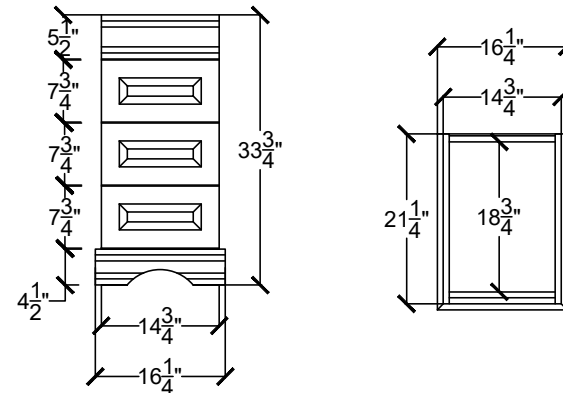
H-ARTS 1522-3D-____-____-____
