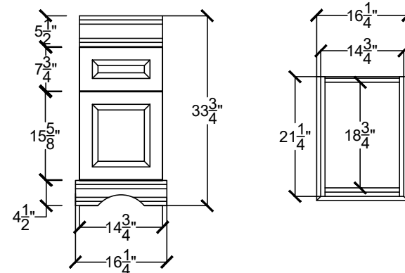
H-ARTS 1522-1D-____-____-____
