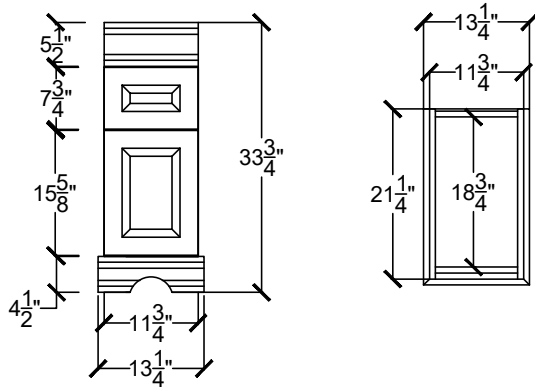
H-ARTS 1222-1D-____-____-____
